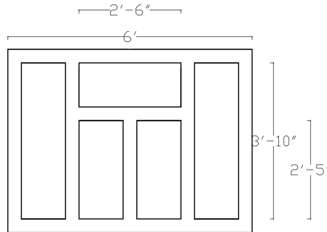
Window Chaukat/Frame
